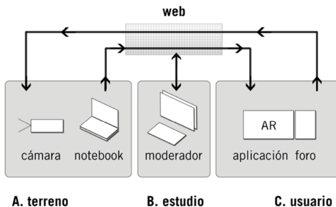
Figura 2. Modelo de flujo de datos.
